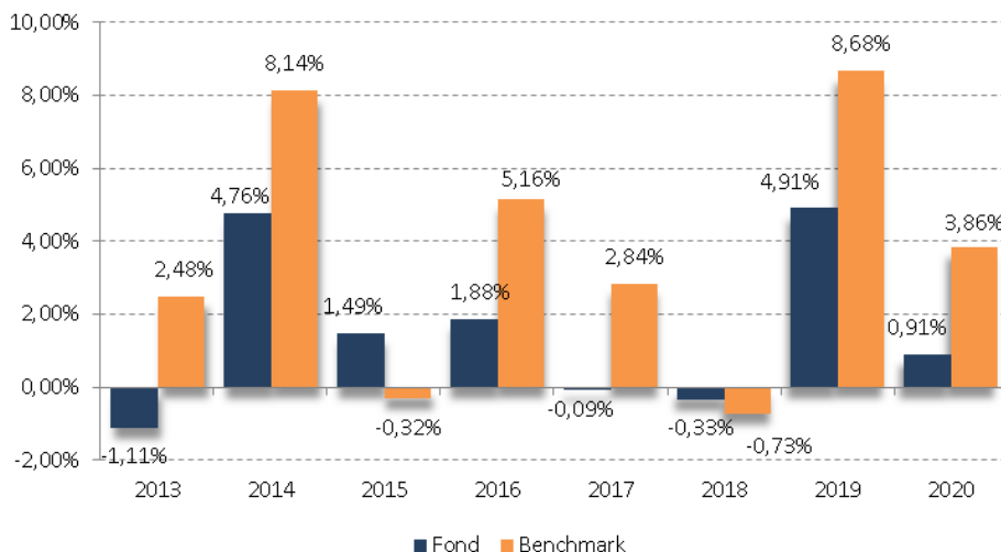
Graf výkonnosti akumulační třídy A (CZ0008473873), počátek 15.1.2013:
